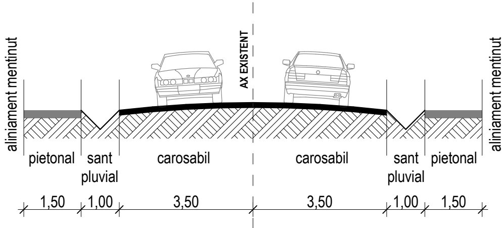
PROFIL MINIM PENTRU STRAZI PRINCIPALE SC. 1:100
