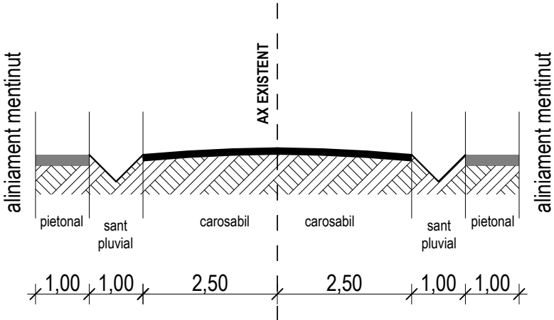
PROFIL MINIM PENTRU STRAZI SECUNDARE SC. 1:100
